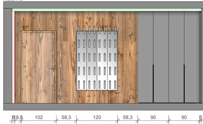
ANSICHT C
