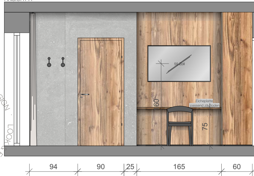
ANSICHT A
