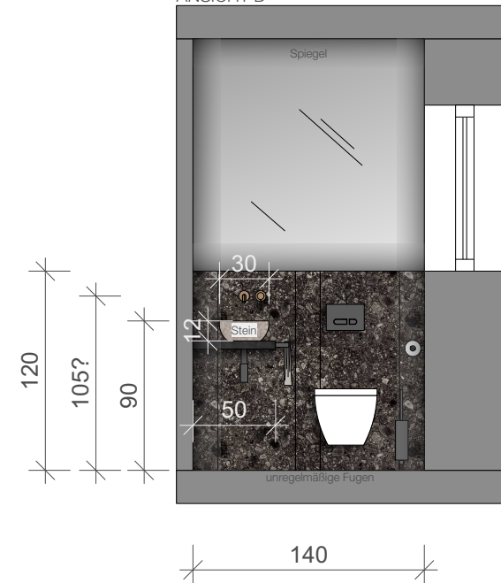
ANSICHT D
