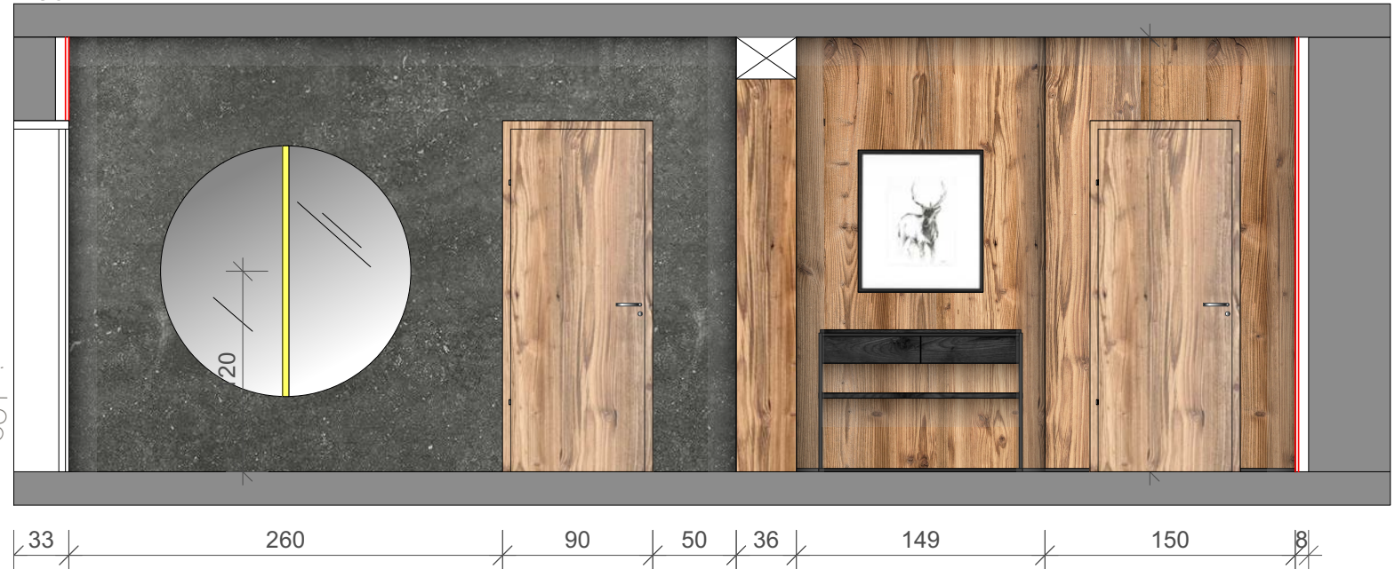
ANSICHT D
