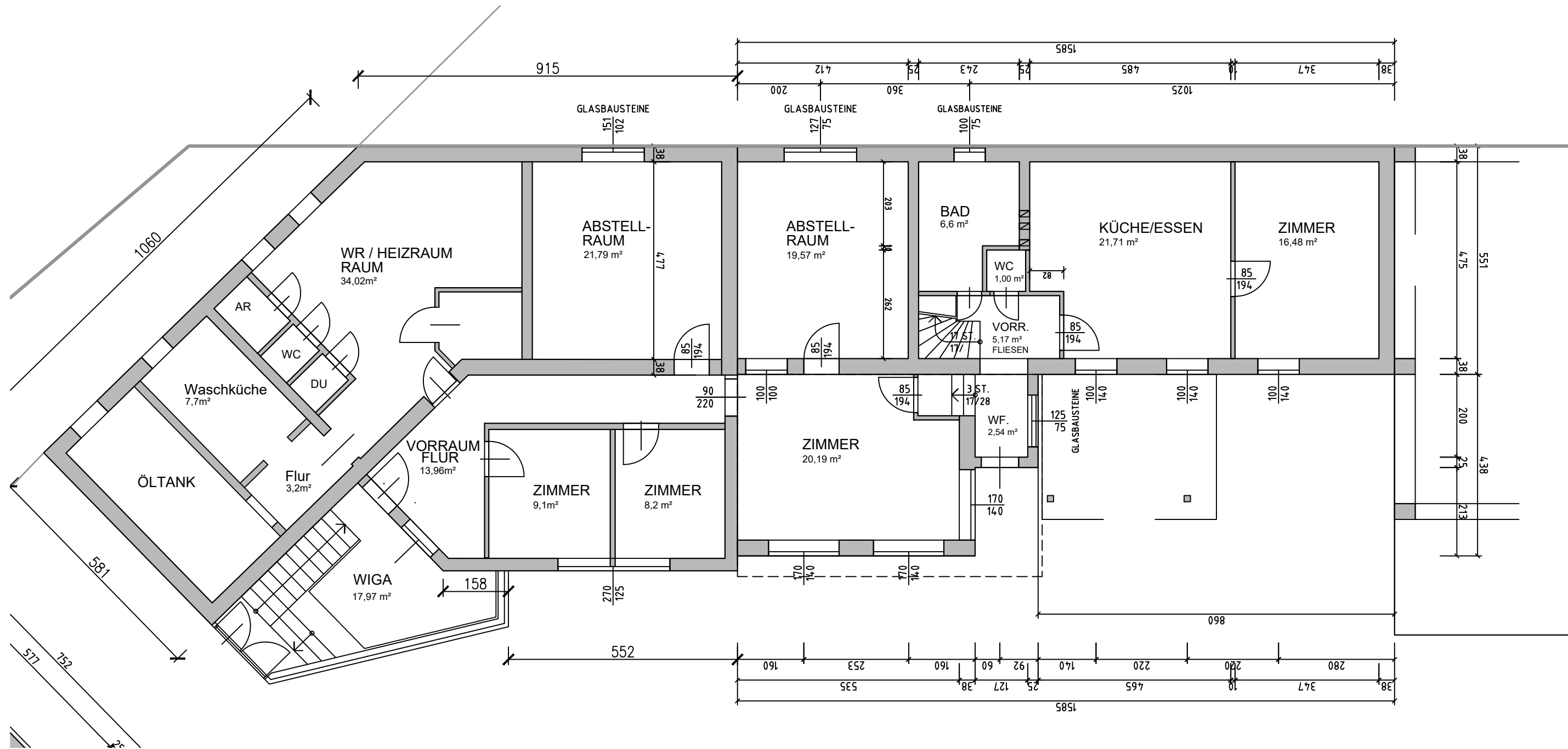
ERDGESCHOSS M 1:100
