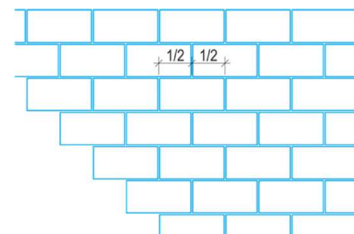
Halbverband
