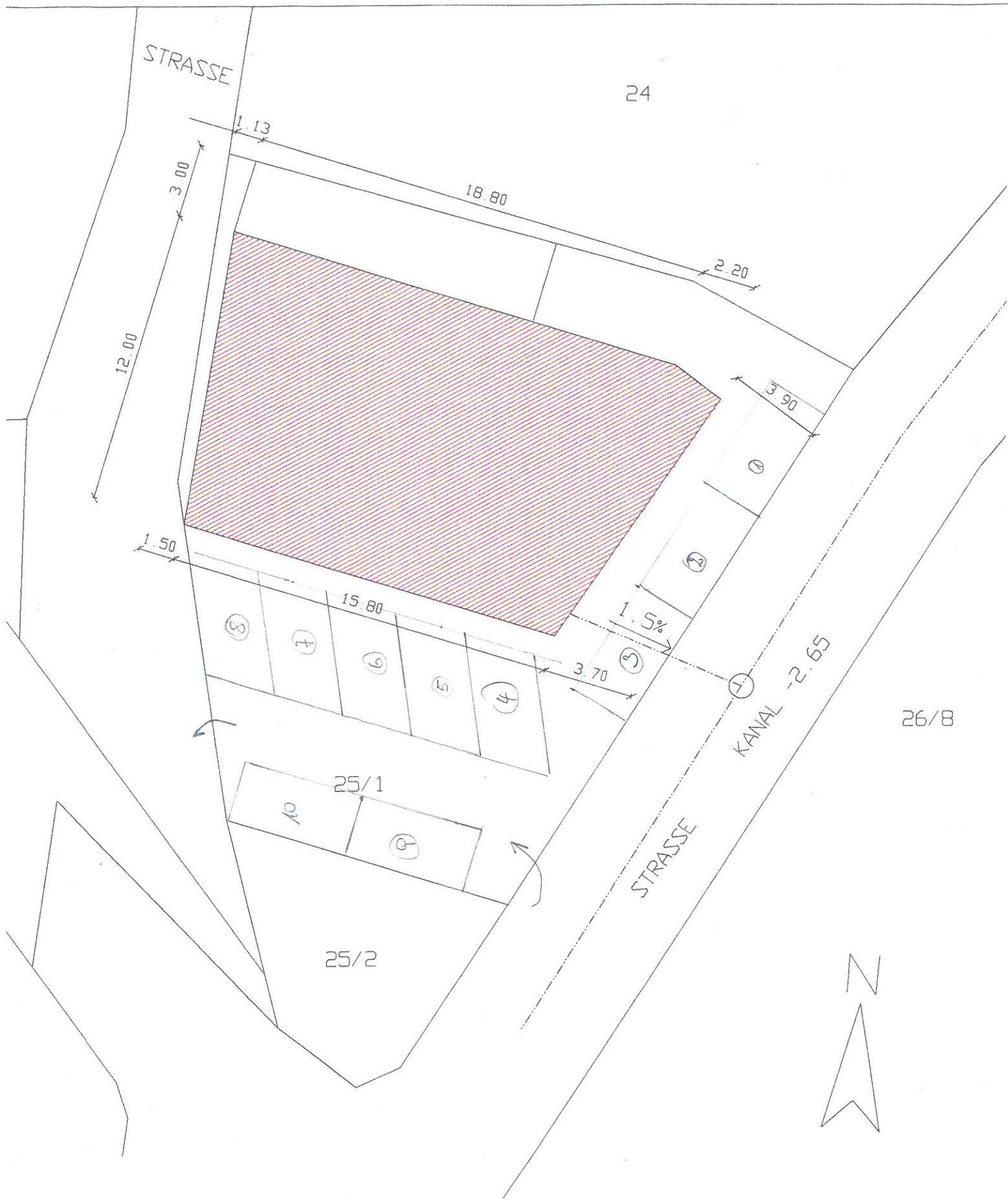
LAGEPLAN M1 : 500
