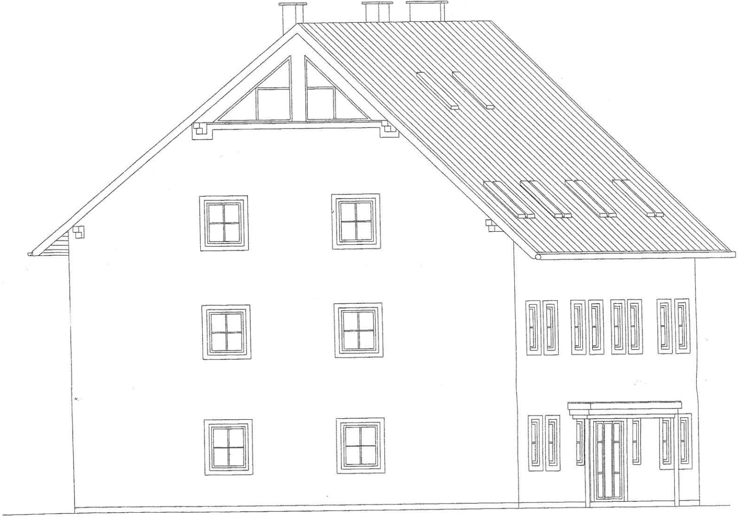
WESTANSICHT
