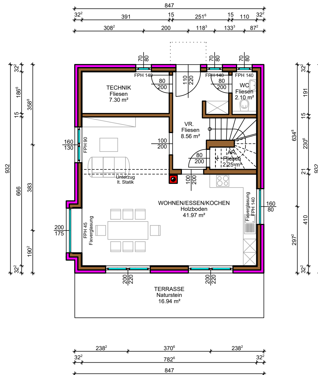
ERDGESCHOSS - M 1:100 Wohnnutzfläche: 62,18 m 2
