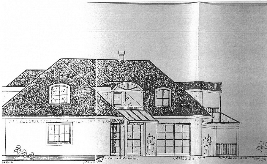
SÜDSICHT 1:100
