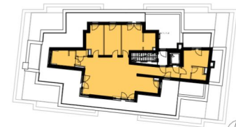
GRUNDRISS STIEGE 5:2. DACHGESCHOSS
