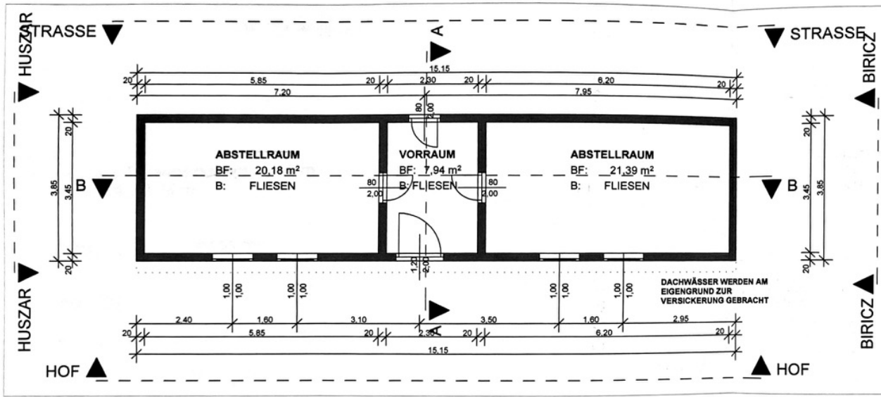
GRUNDRISS ERDGESCHOSS M 1:100
