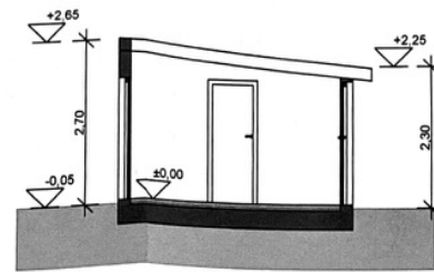
SCHNITT A-A M 1:100
